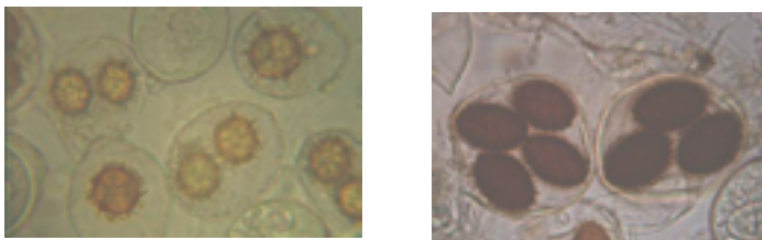
Fig. 2.6 Diverse tipologie di ascospore
