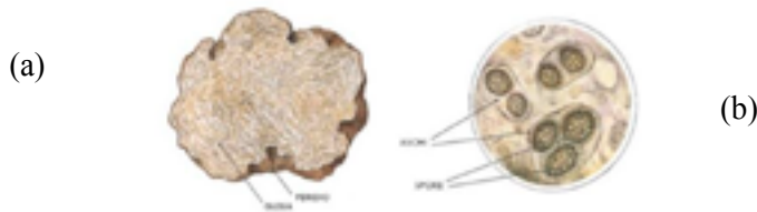
Fig. 2.5 – Sezione di ascoma o “corpo fruttifero” con gleba (a); strutture riproduttive cioè aschi con ascospore (b)
